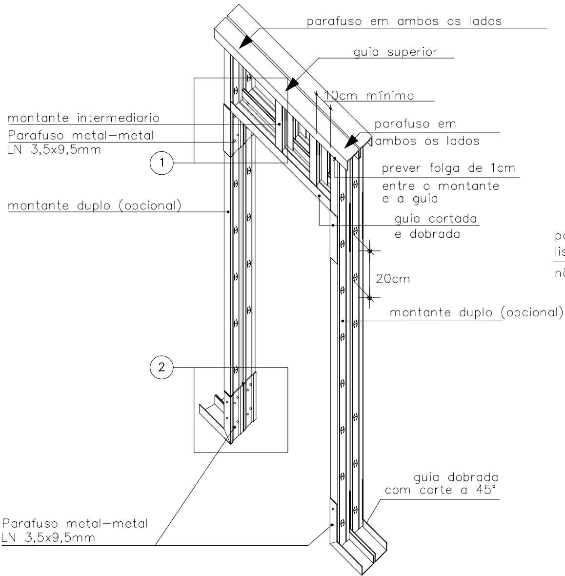
1 PERSPECTIVA SEM ESCALA
