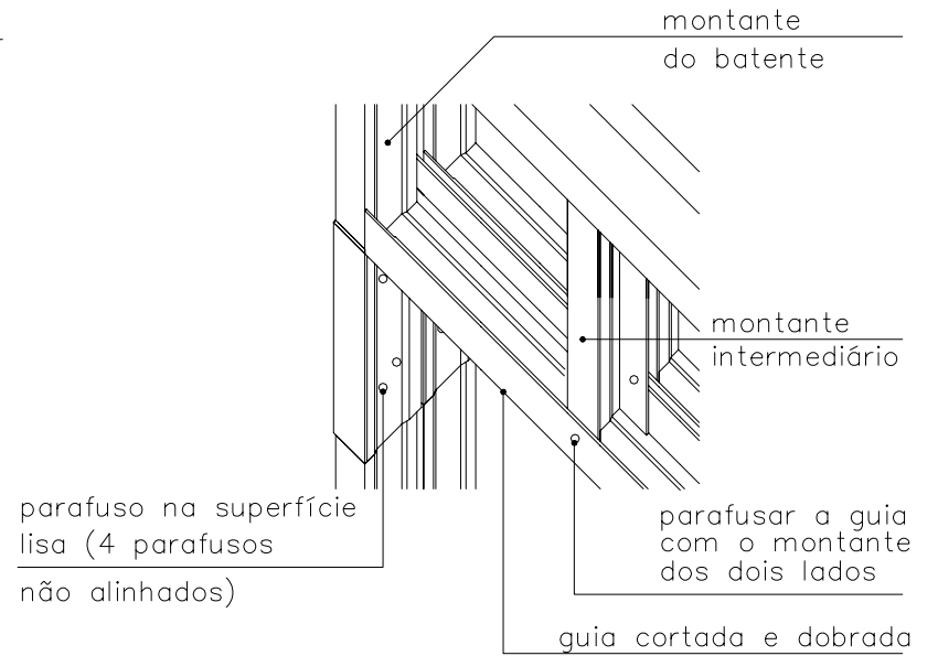
2 DETALHE 1 SEM ESCALA
