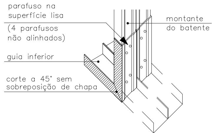
3 DETALHE 2 SEM ESCALA
