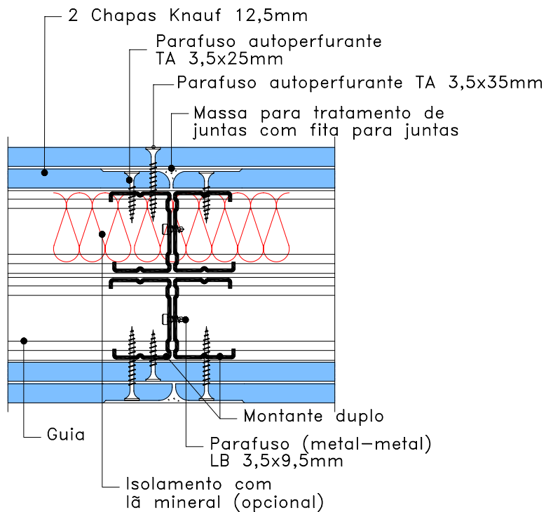
DETALHE – JUNTA DE CHAPAS ESTRUTURA DUPLA – W115 SEM ESCALA
