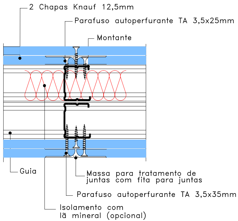
DETALHE – JUNTA DE CHAPAS ESTRUTURA SIMPLES – W115 SEM ESCALA
