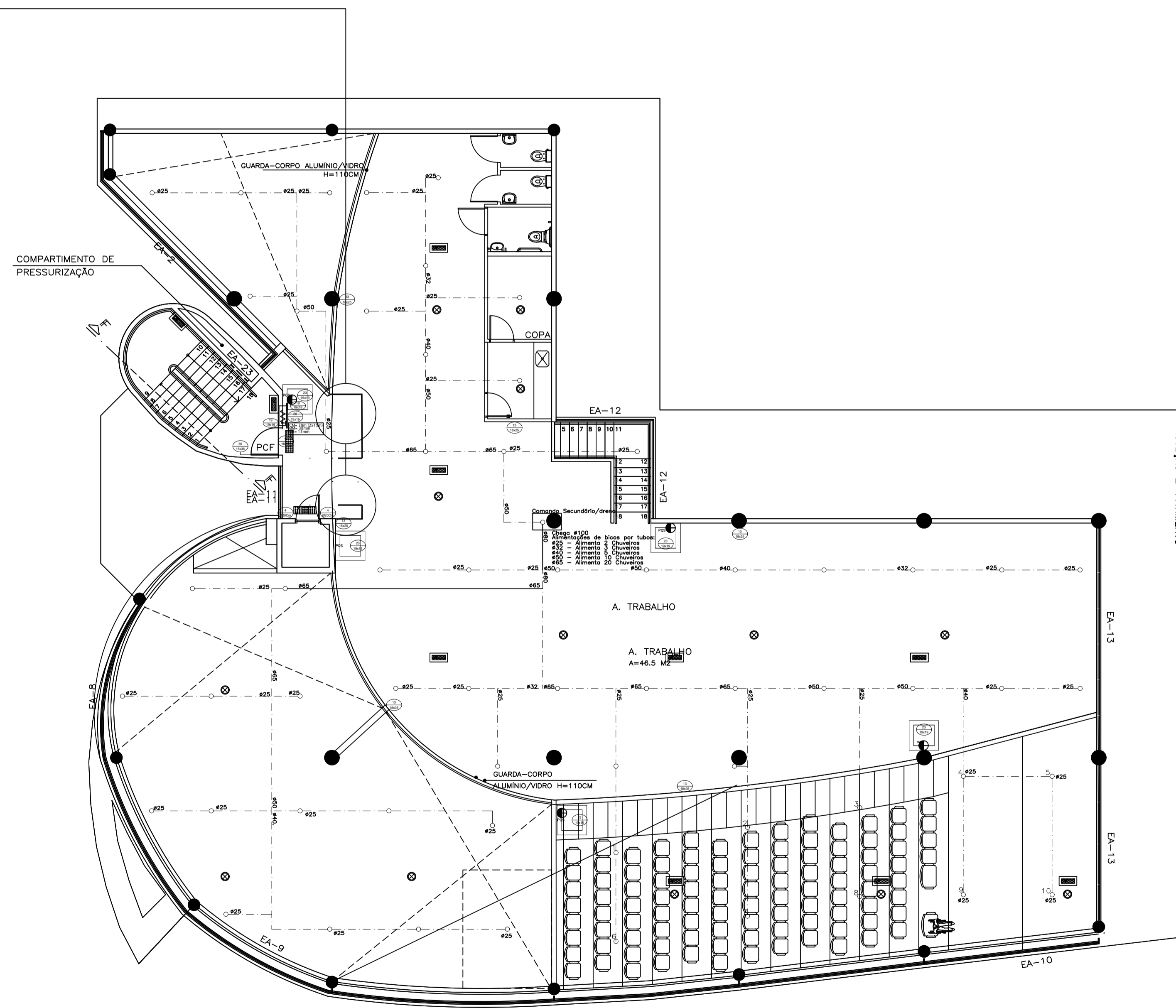
PLANTA MEZZANINO Esc.: 1\100
