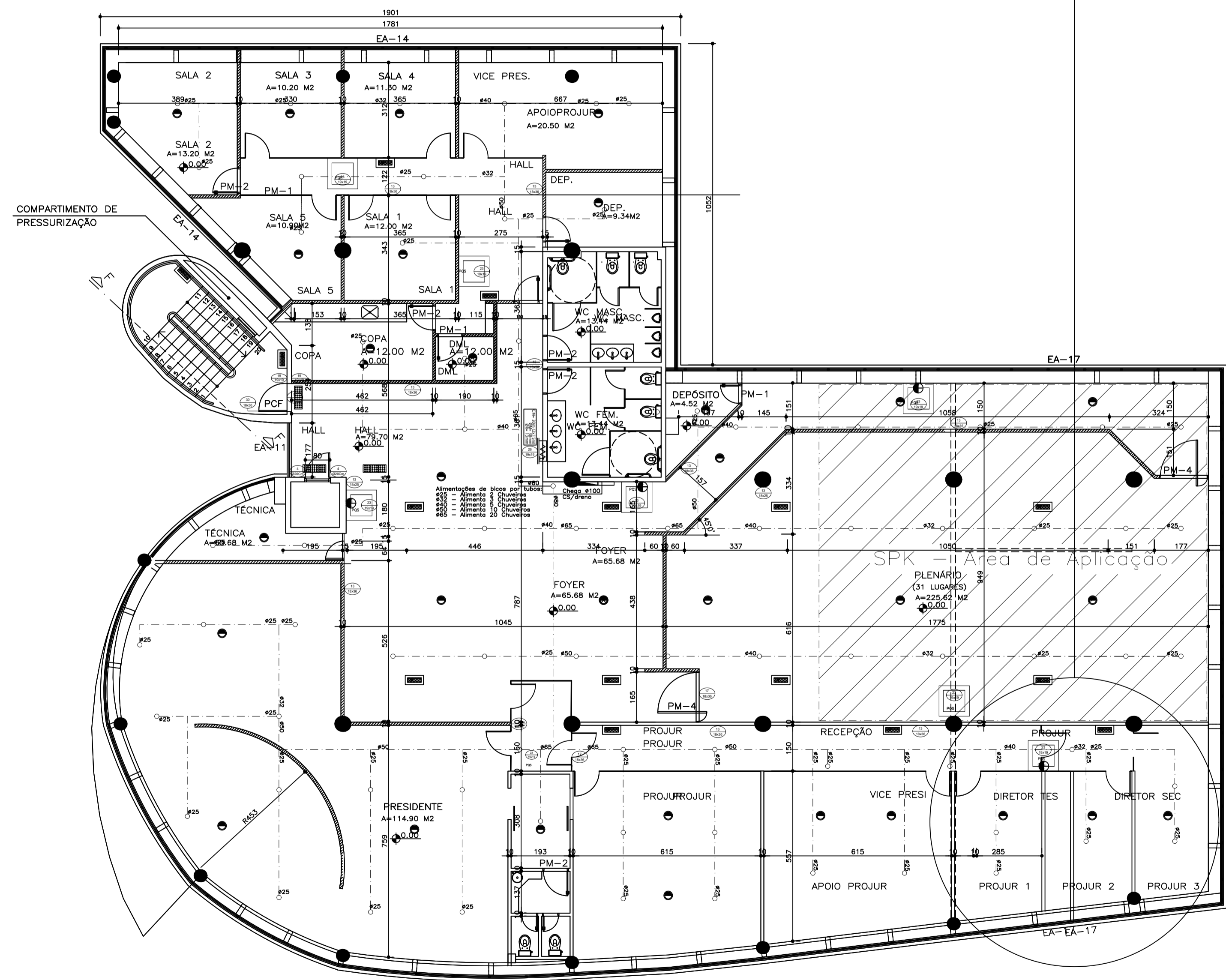
PLANTA 4º PAVIMENTO ESC: 1/100
