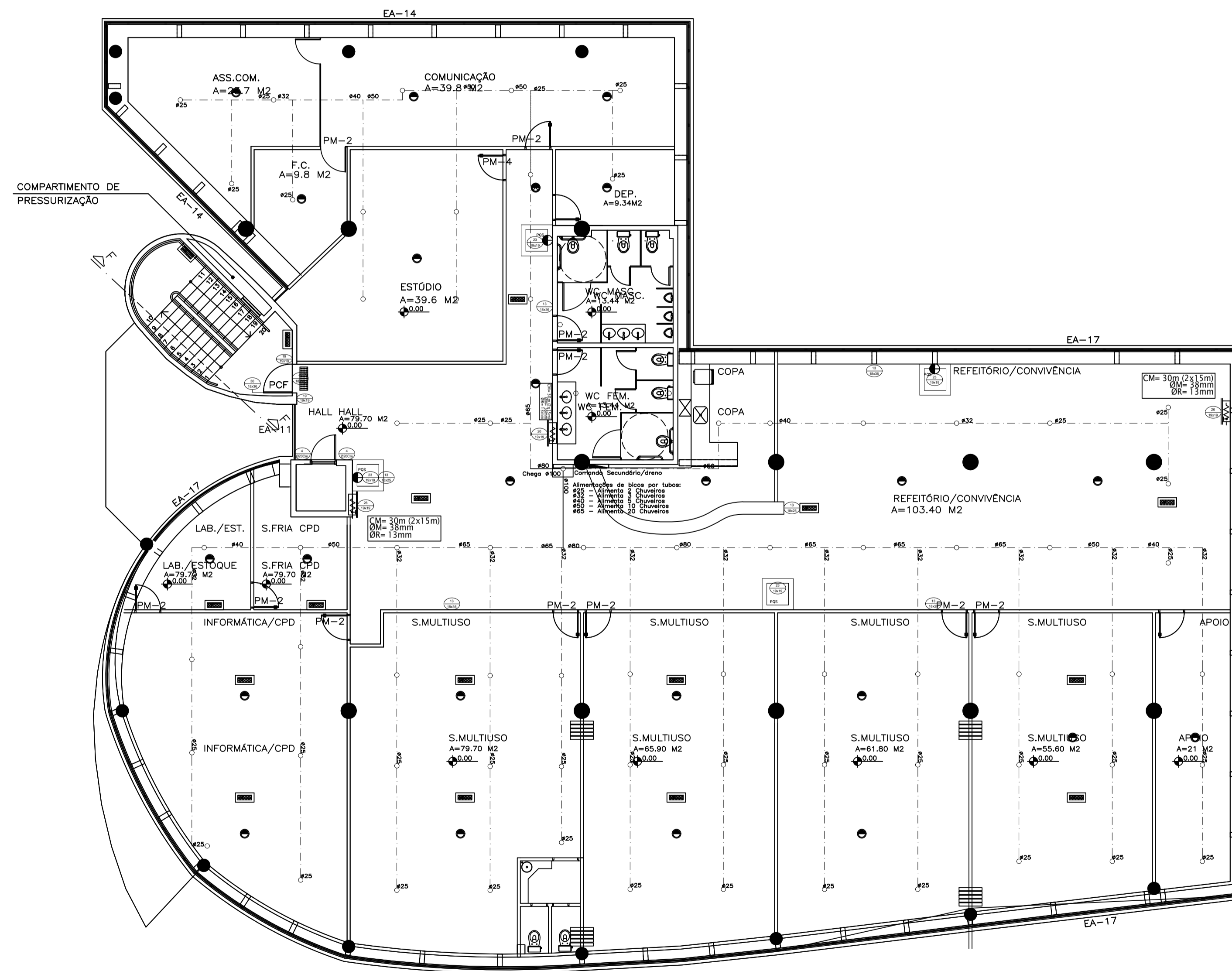
PLANTA 3º FAVAMENTO ESC.: 1/100
