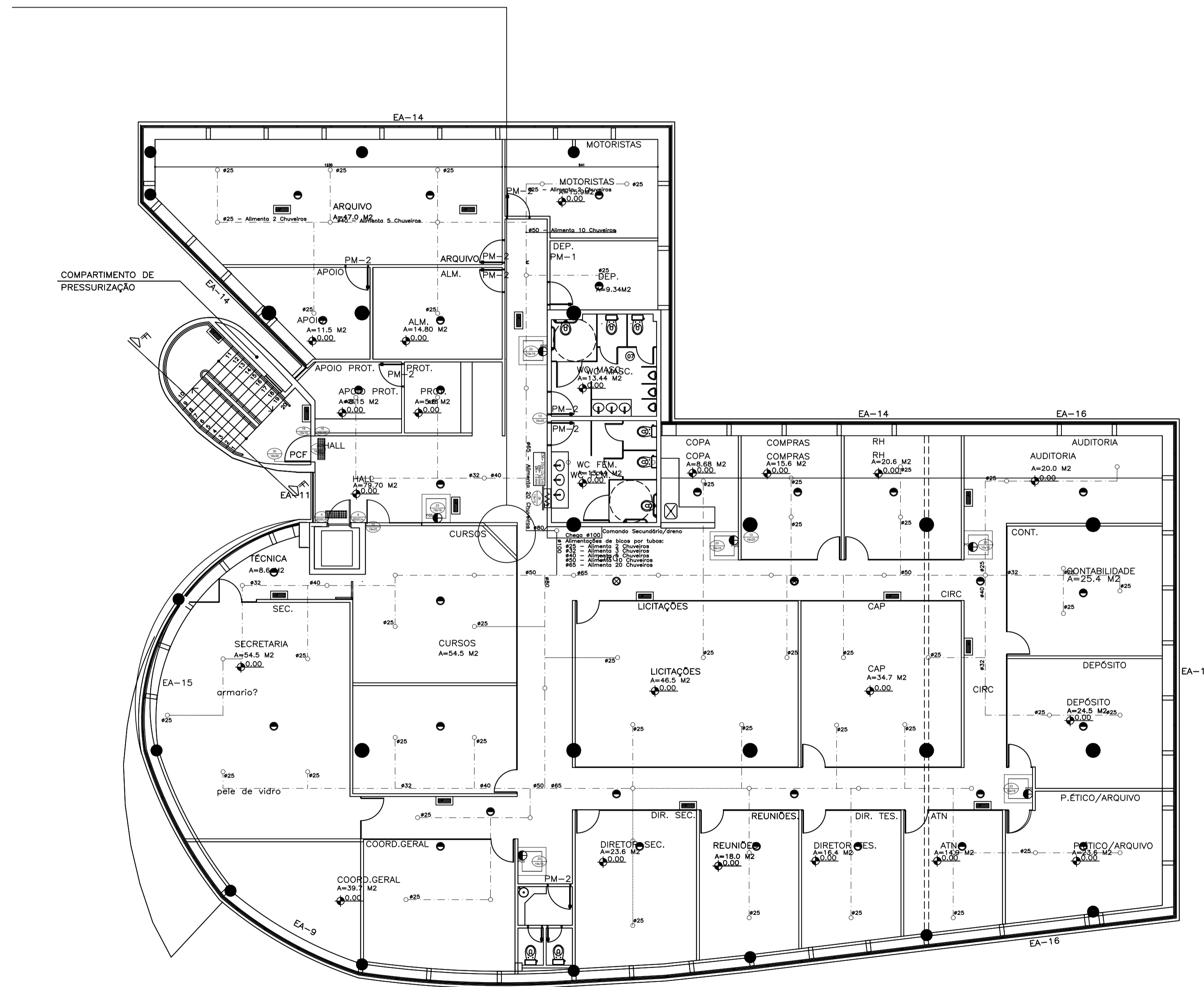
PLANTA 2º FAVAMENTO ESC: 1/100
