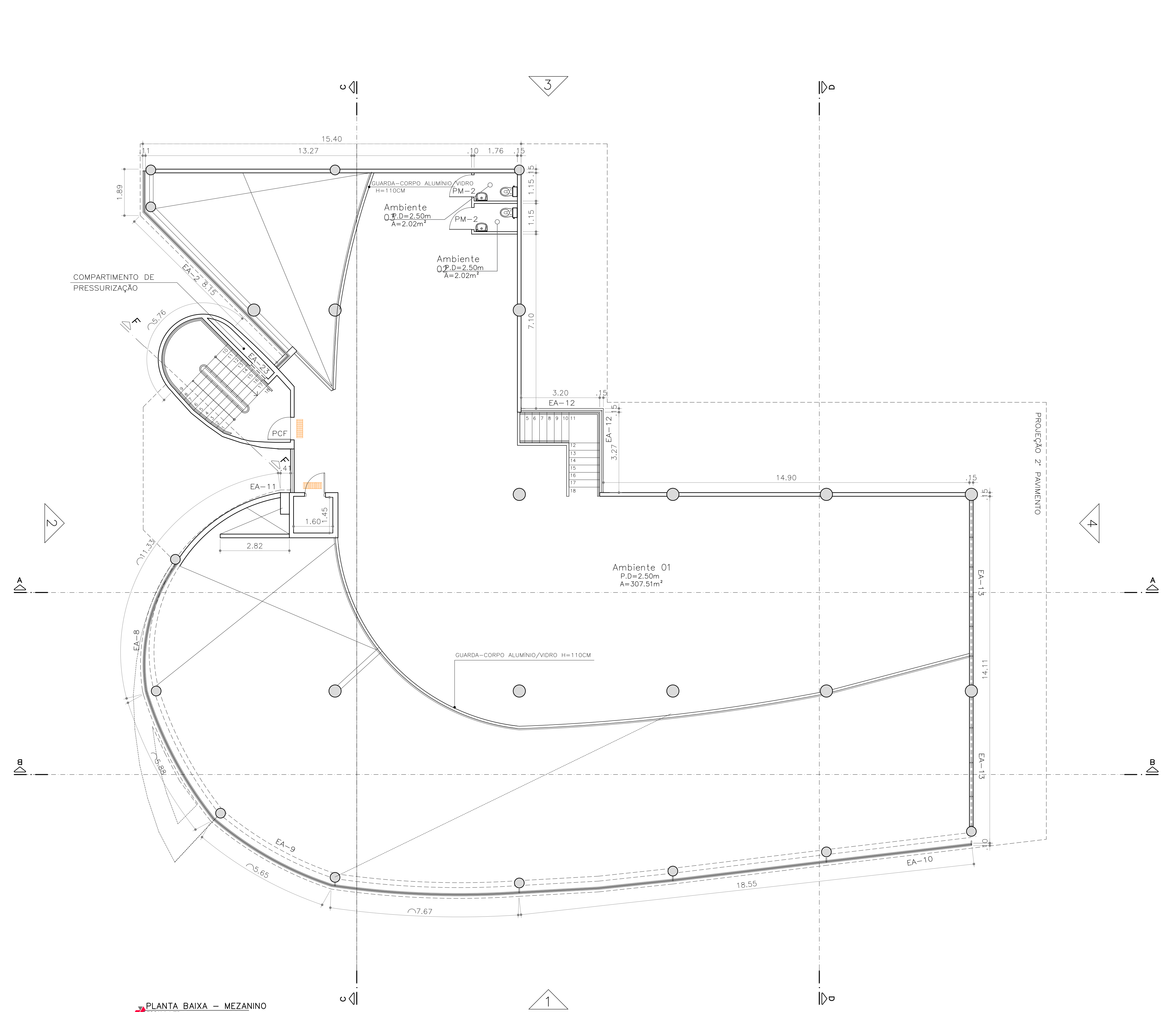
PLANTA BAIXA - MEZANINO ESCALA 1/75
