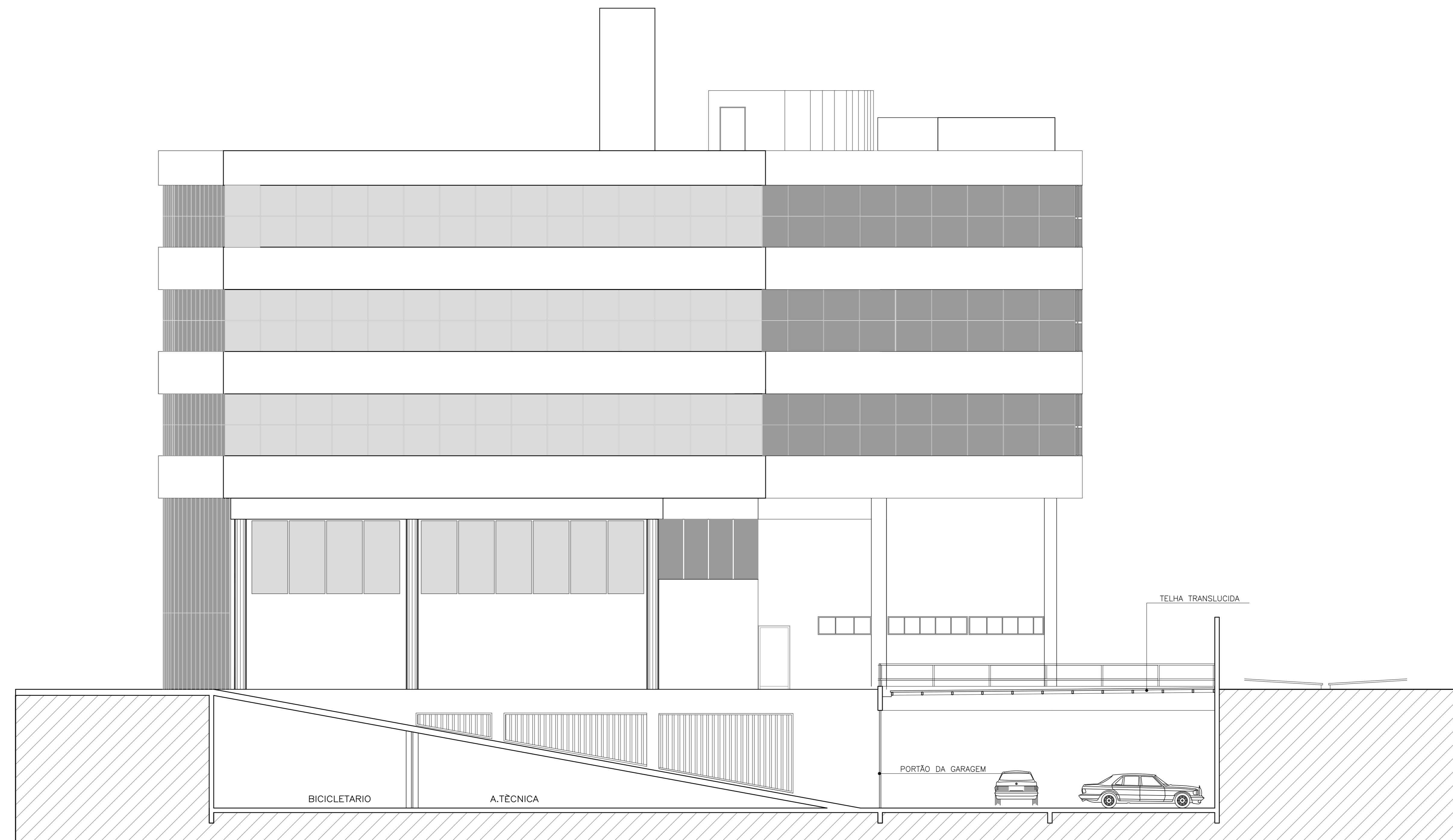
ELEVAÇÃO 04 ESC.: 1\75
