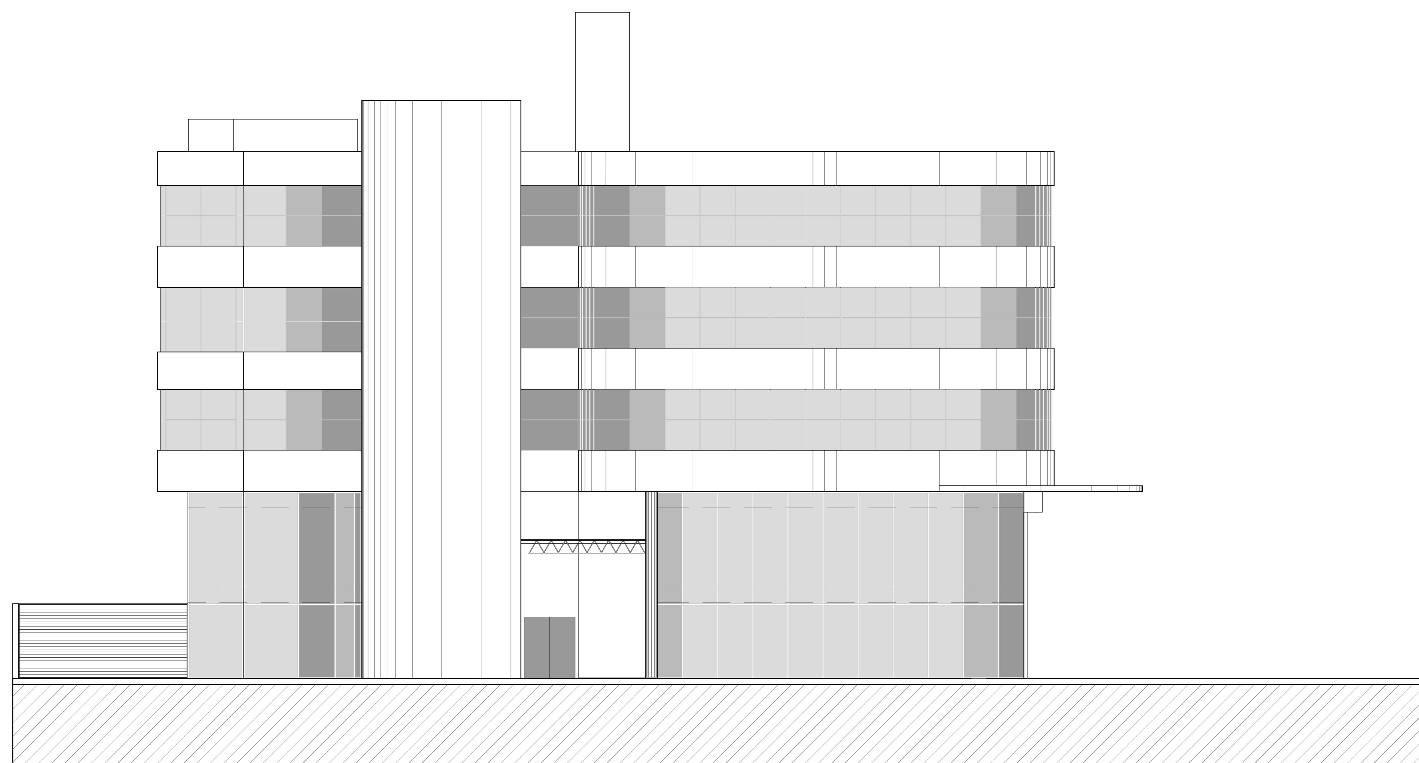
ELEVAÇÃO 02 ESC.:1\,75
