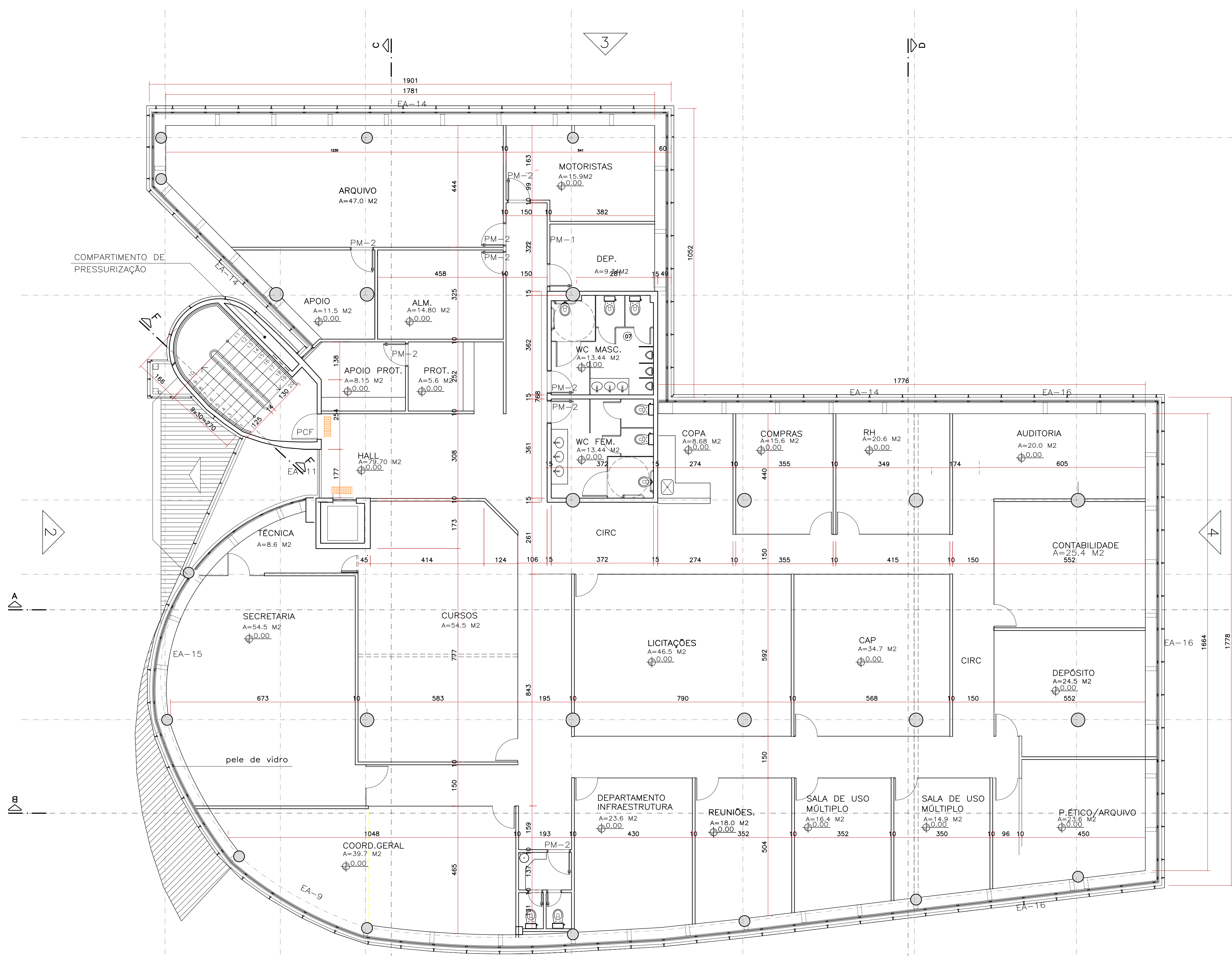
PLANTA 2 PAVIMENTO ESC:1/75
