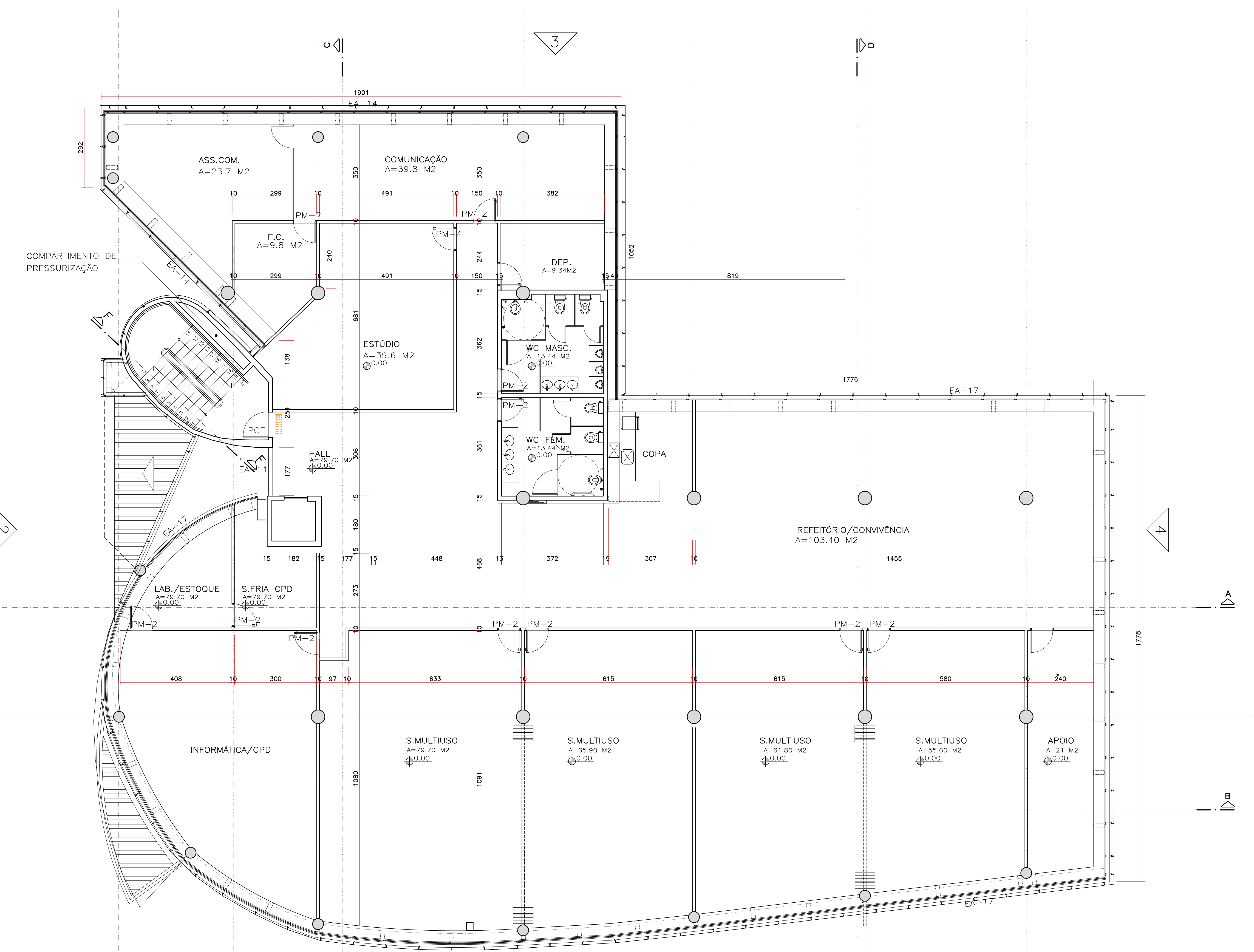
PLANTA 3 PAVIMENTO ESC:1/75
