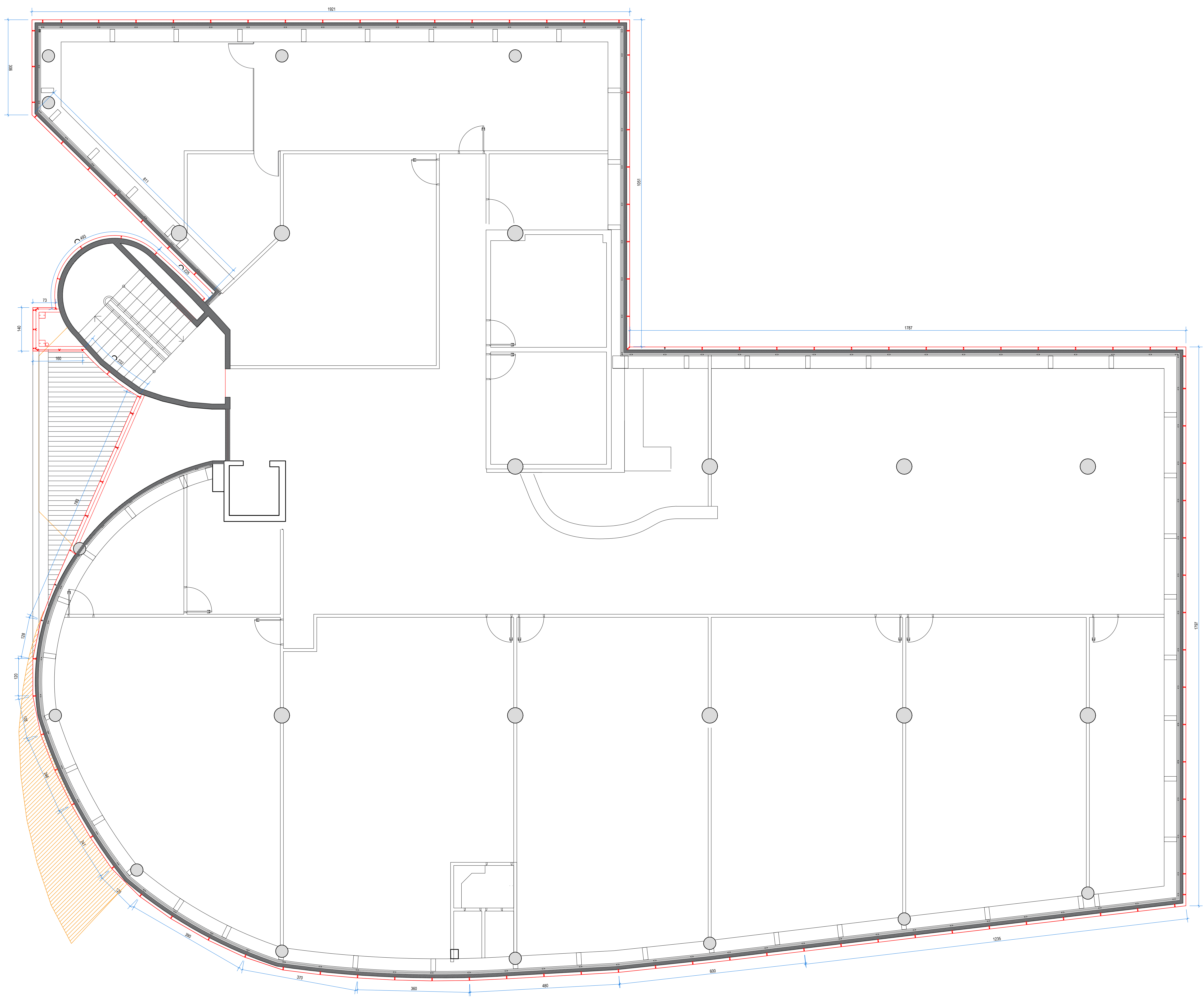
PLANTA 3 PAVIMENTO ESC.:1\100
