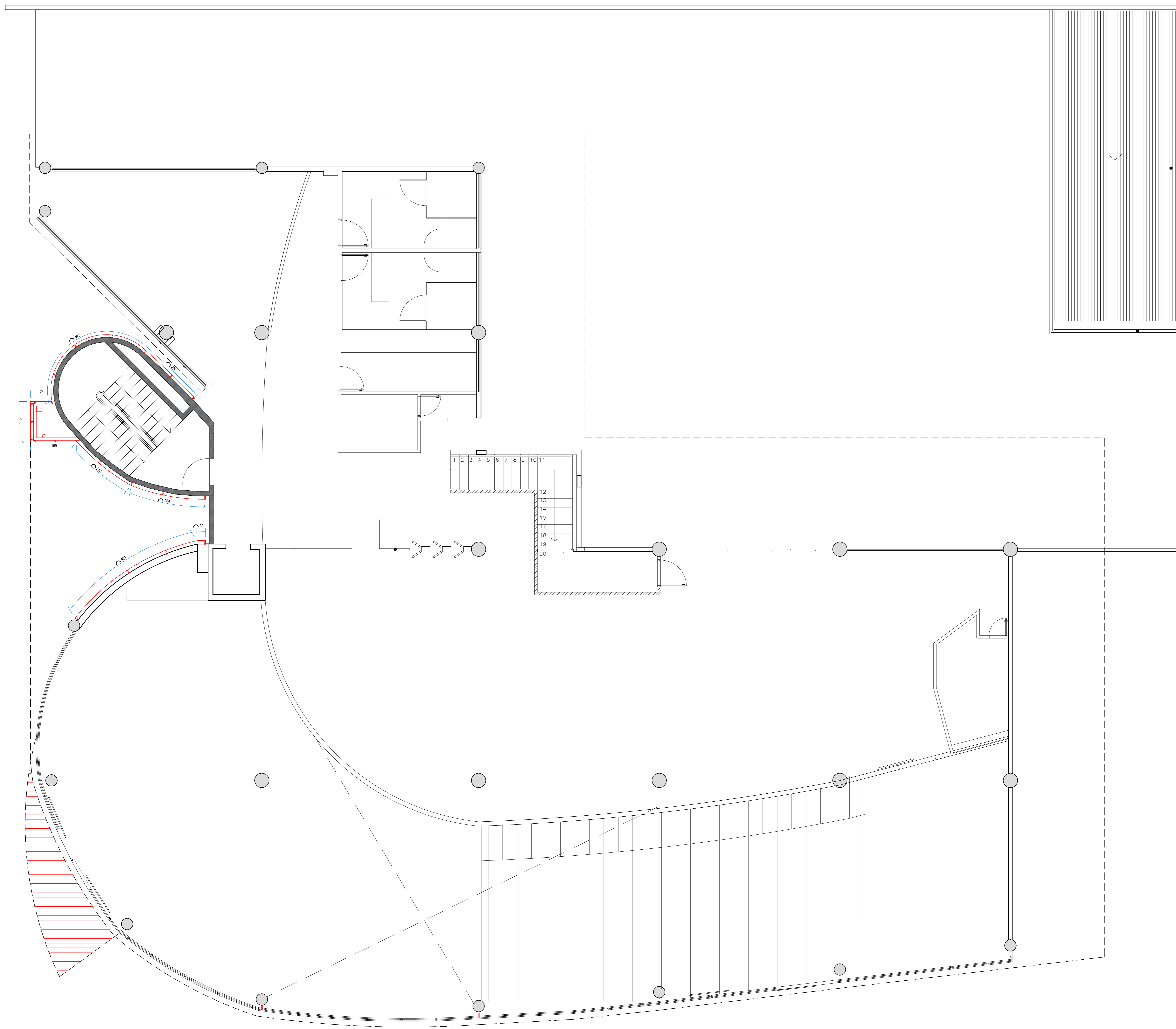
PLANTA TÉRREO ESC.: 1\100
