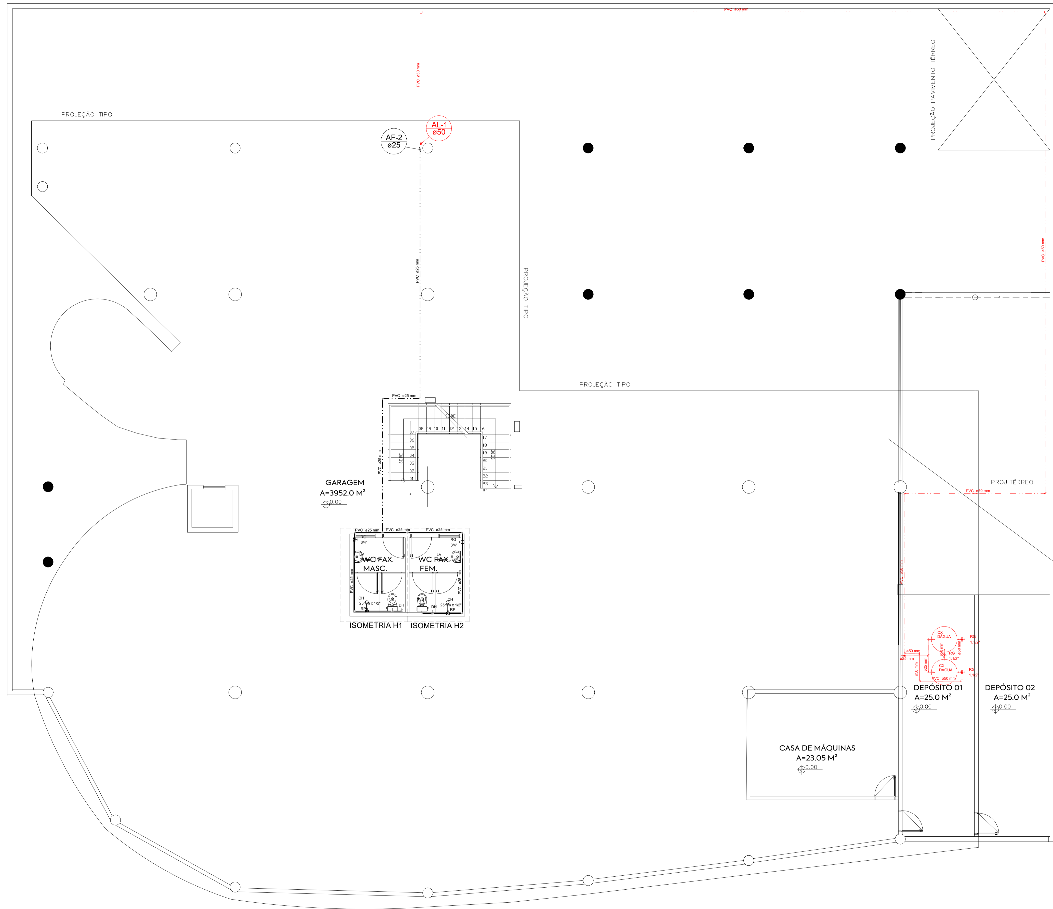
PLANTA BAIXA - HIDRO SUBSOLO ESCALA 1/75
